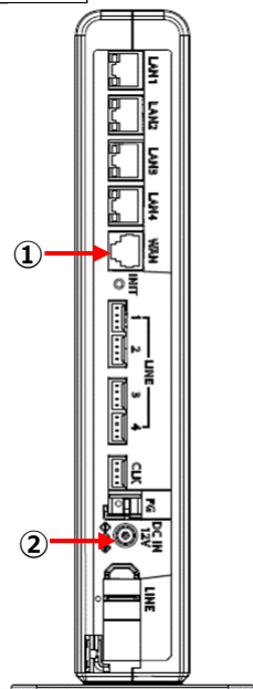
本装置 SG2000is4/is8 背面図
